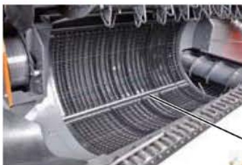
こぎ胴受アミ
