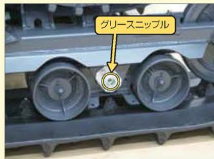
2) 転輪揺動軸部分(左右各1箇所)
